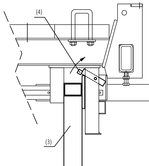
Elevation E
