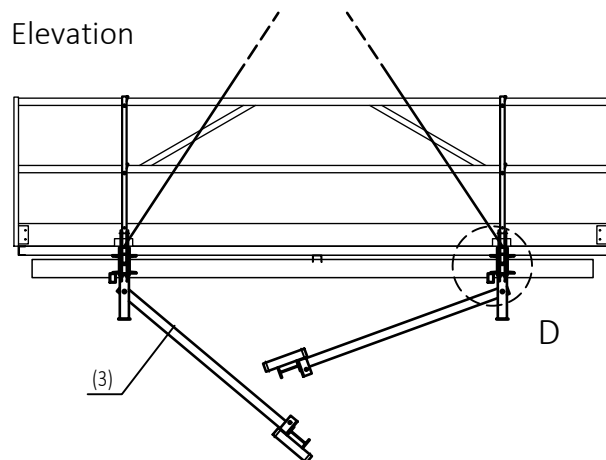
Elevation E
