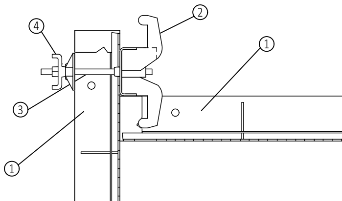
Detal A : połączenie narożne
