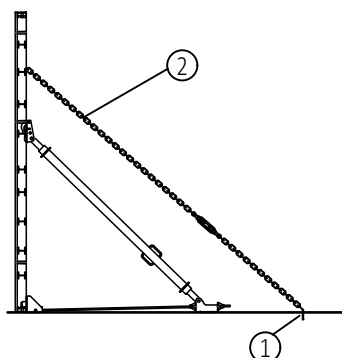
Łańcuch napinający
