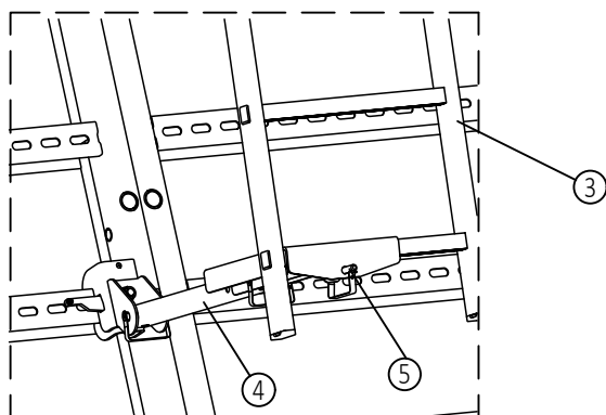
Detal B
