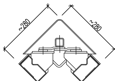
Przykładowy zarys w pozycji rozszalowującej
