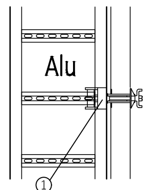
Przekrój 1-1
