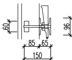
Przekrój 3-3
