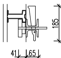
Przekrój 3-3
