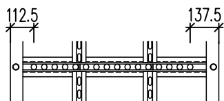
Widok listwy otworowej AET typowa
