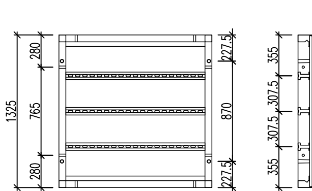
Przekrój
