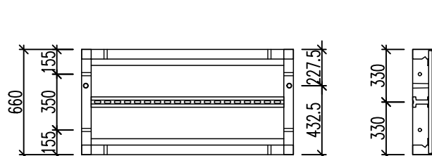
Przekrój
