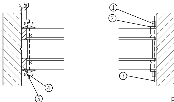
Widok A-A
