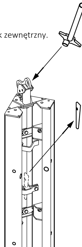
Ilustracja bez zamocowanej płyty szalunkowej NOEtop
