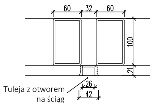
Przekrój - zintegrowanego pasa mocującego z otworem na ściąg
