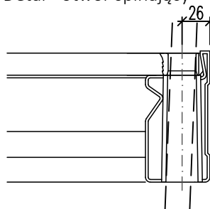
Detal - otwór spinający
