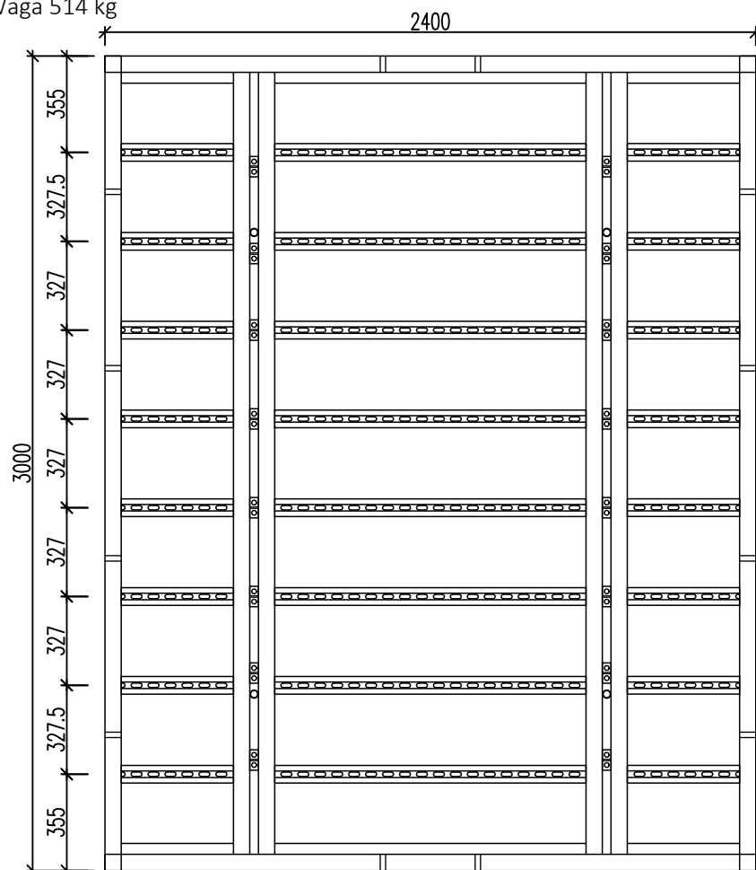
Przekrój poprzeczny
