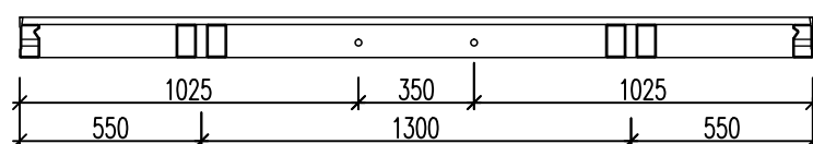
Przekrój poprzeczny
