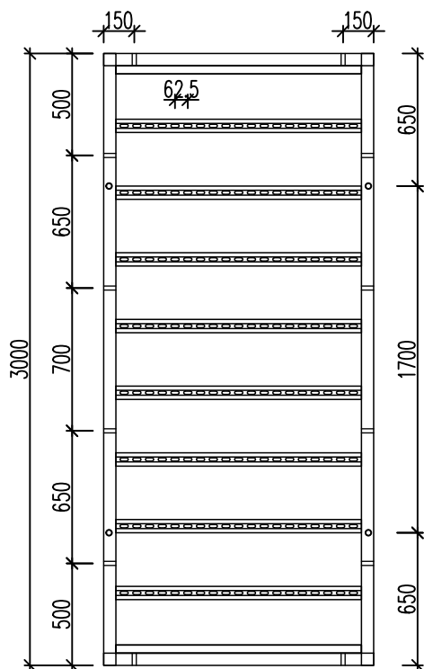
Widok
