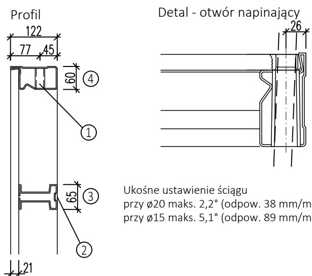
Przekrój
