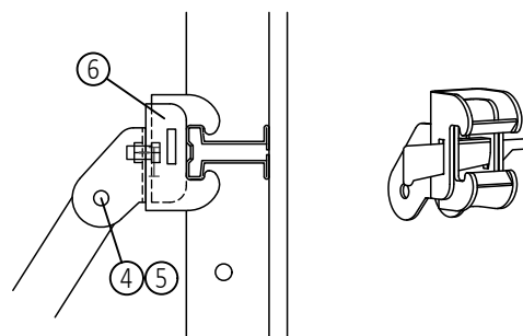
Detal A
