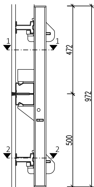
Przekrój 1-1
