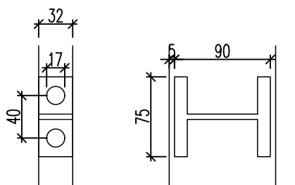
Detal - element dystansowy w zintegrowanym pasie mocującym
