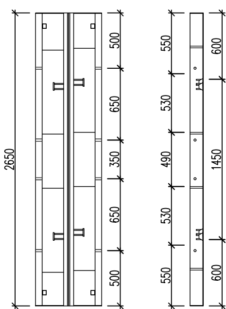
Wysokość 2650 mm
