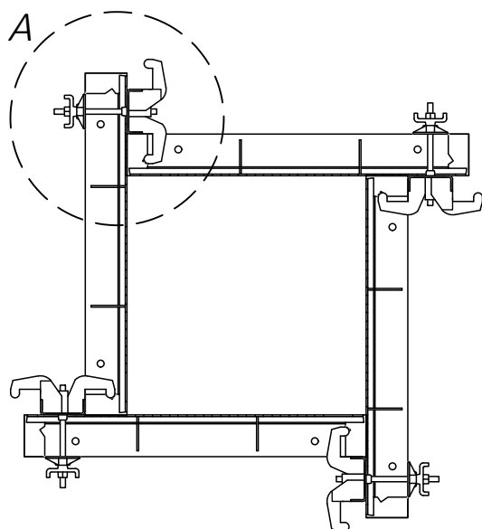
Detal A : połączenie narożne
