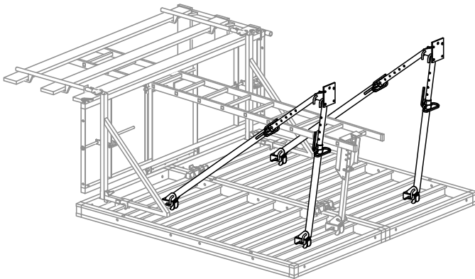
Pierwszy element z dwoma zastrzałami
