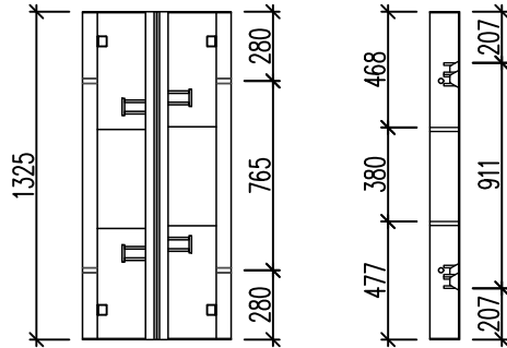
Wysokość 1325 mm
