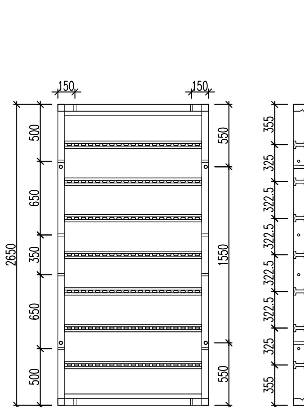
Przekrój
