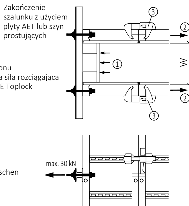
Zakończenie ściany
