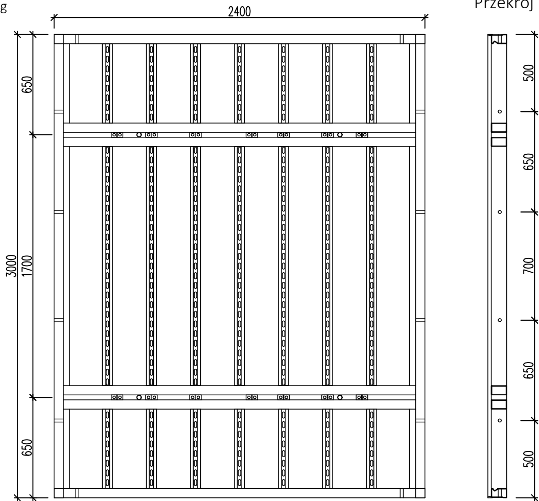
Przekrój poprzeczny
