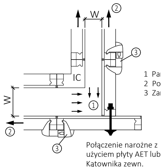
Zewnątrz naroża
