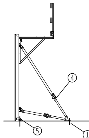
Szalunek jednostronny
