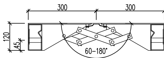
Przekrój
