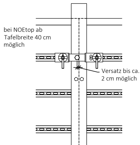
NOEtop Tafel stehend Befestigung am Tafelstoß
