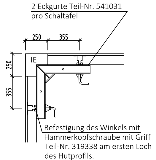
Detail Befestigung der Eckgurte
