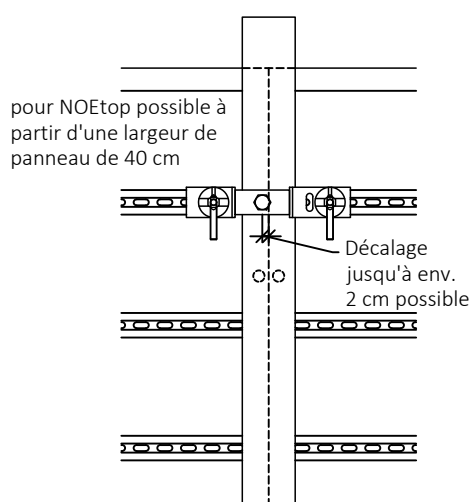
Fixation à la jonction de panneau
