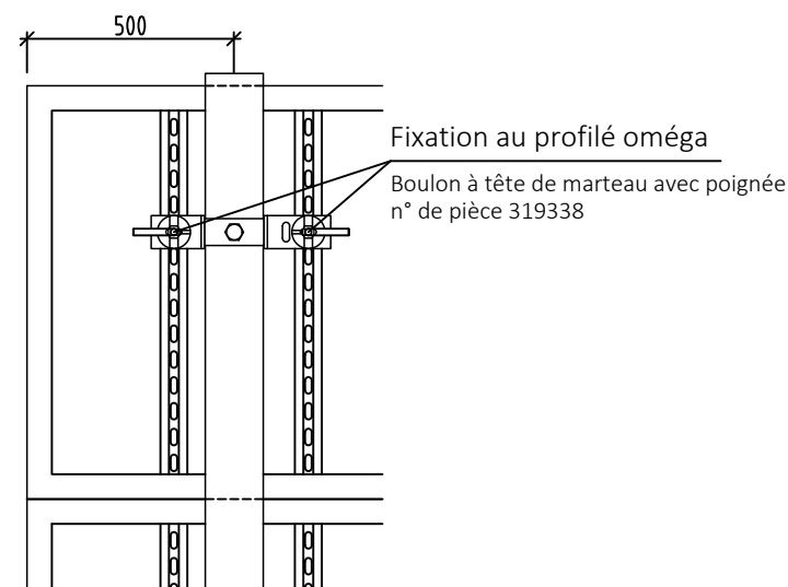
NOEtop panneau couché
