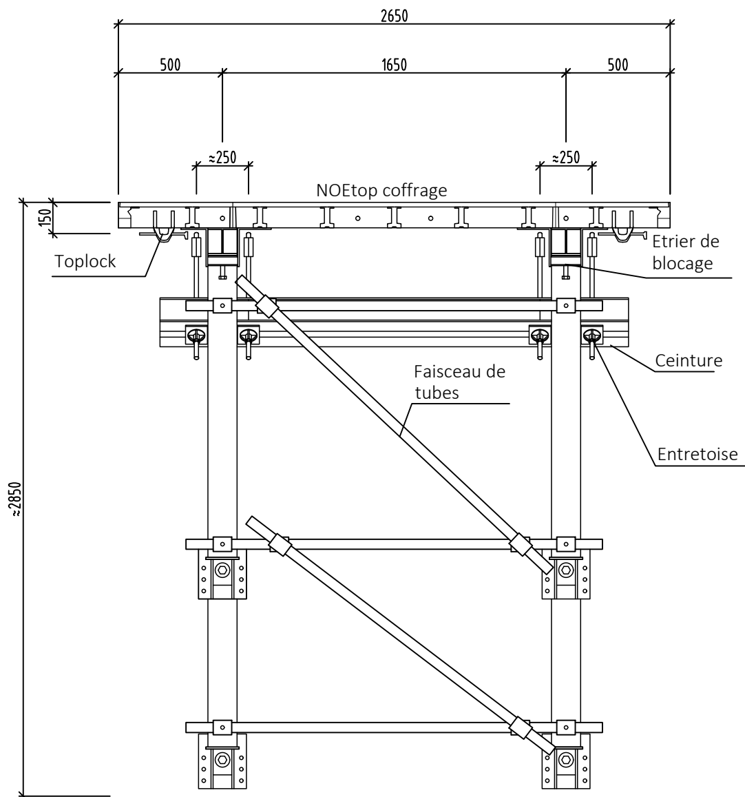
Ceinture N° de pièce 541030 Poids 107 kg
