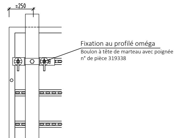
Fixation au panneau
