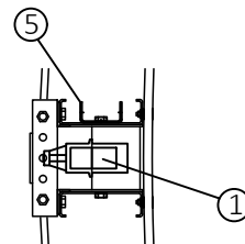
Coupe élément extérieur à travers paire de poutrelles
