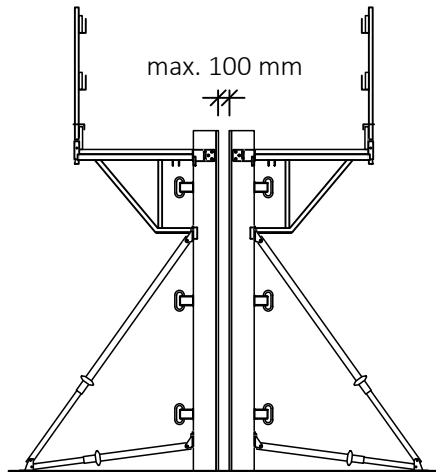
Schalung doppelseitig
