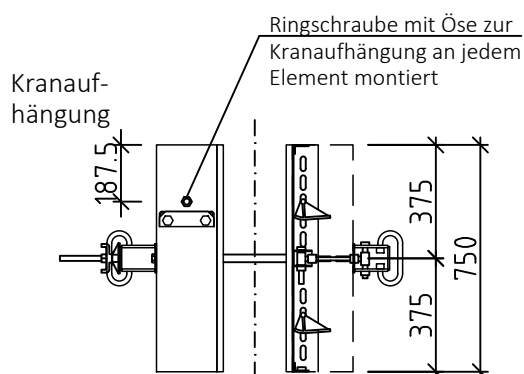
Aufstockelement 750 mm
