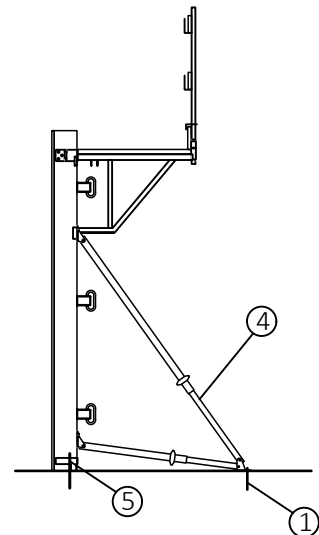
Schalung einseitig
